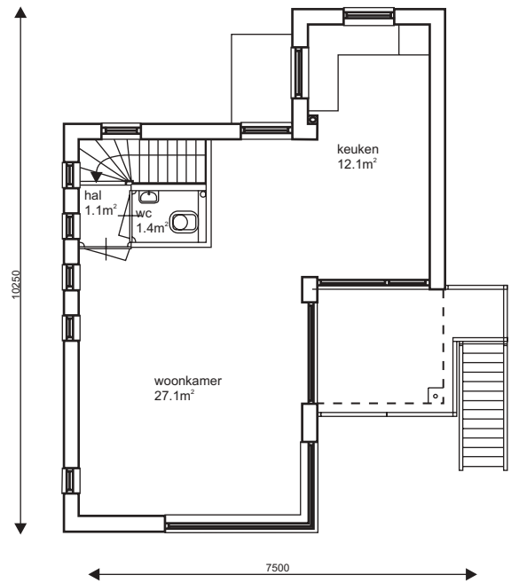
Plattegrond verdieping
